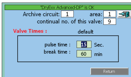
fig. 7.13
