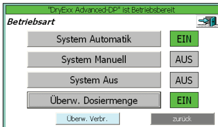
Abb. 7.20
